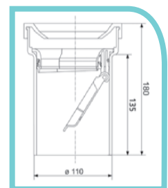
Art. Nr. 3759028 PE wandclosetaansluitstuk recht d110
