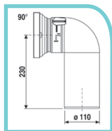
Art. Nr. 3759032 PP staand closetaansluitstuk bocht d110 - 90°
