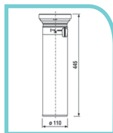
Art. Nr. 3759033 PP staand closetaansluitstuk recht d110
