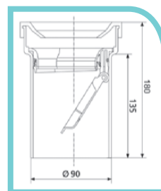
Art. Nr. 3759034 PE wandclosetaansluitstuk recht d90
